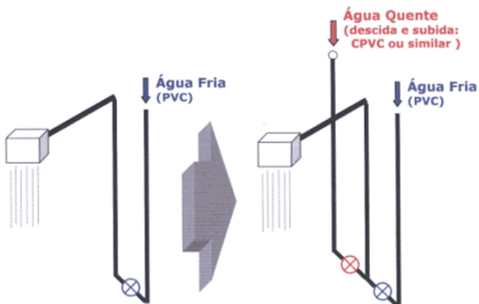
Figura 04: Tubulação de espera para água quente.
