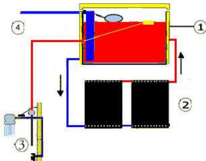
Figura 1. Representação de um ASBC residencial.
